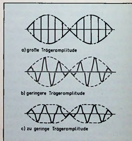
Bild 8.2: Ringmodulator-Ausgangssignale
