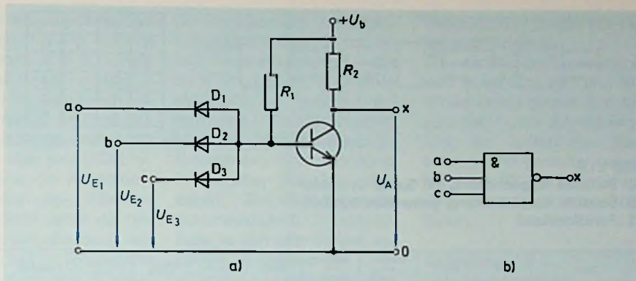
Bild 1.1.7: Das NAND-Glied ist eine Kombination aus einem UND-Glied und NICHT-Glied
