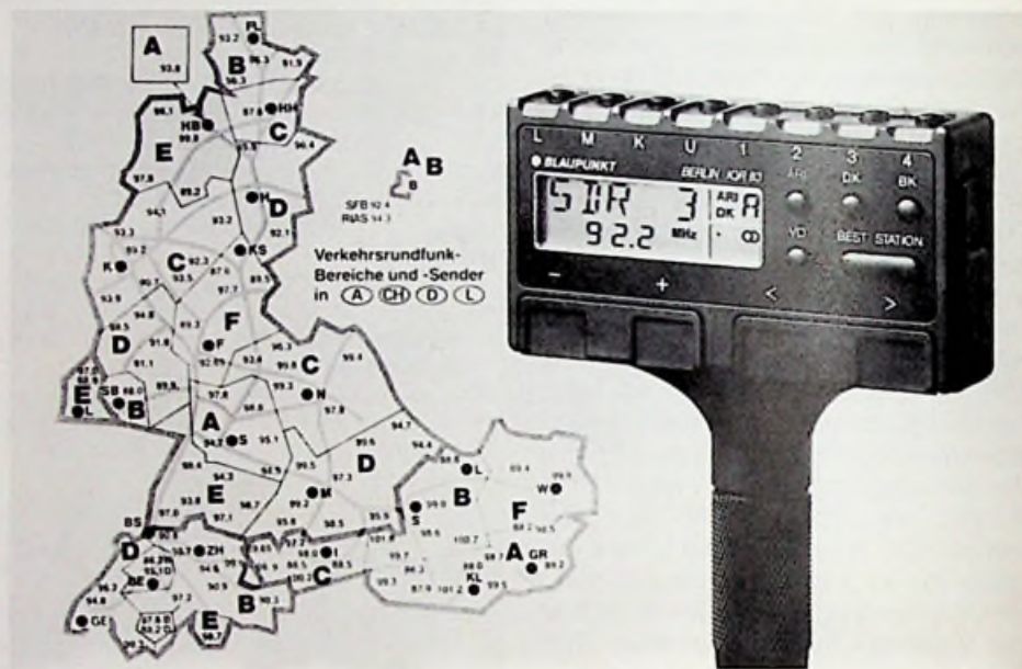
Bild 1: Der Bedienteil des neuen Autoradios IQR 83 mit viel Komfort (Blaupunkt-Pressbild)
