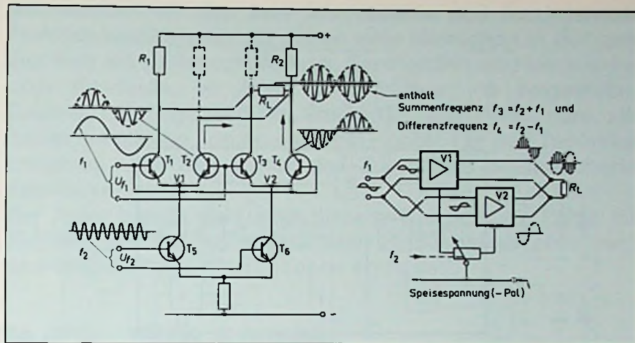
Bild 7.1: Arbeitsprinzip als Mischer
