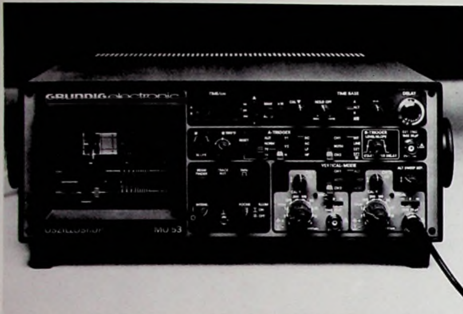
Bild 3: Front des neuen 50-MHz-Oszilloskops MO 53 von Grundig
