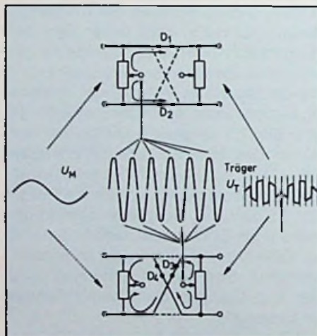
Bild 8.1: Spannungen am Ringmodulator
